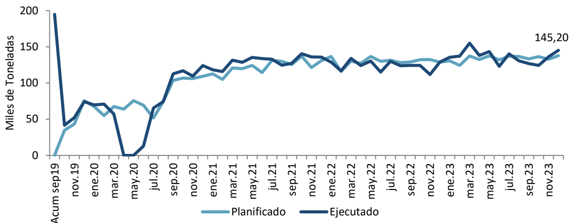
Figura 4. Cantidad de mena explotada Mina Fruta del Norte En miles de toneladas, 2019-2023
